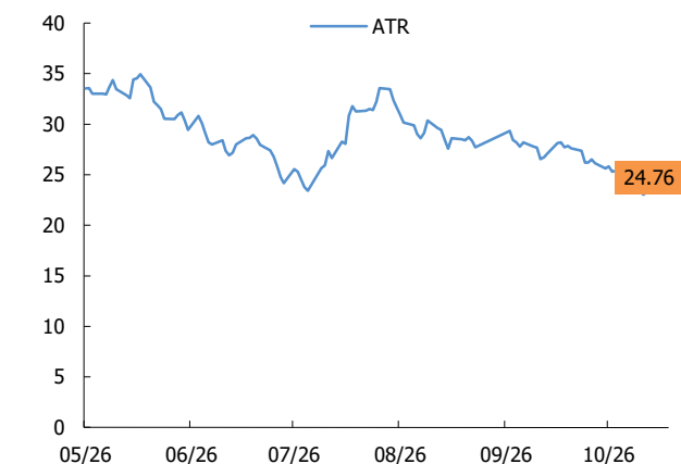
Hình 4. Chỉ báo dao động (ATR) - VNIndex
